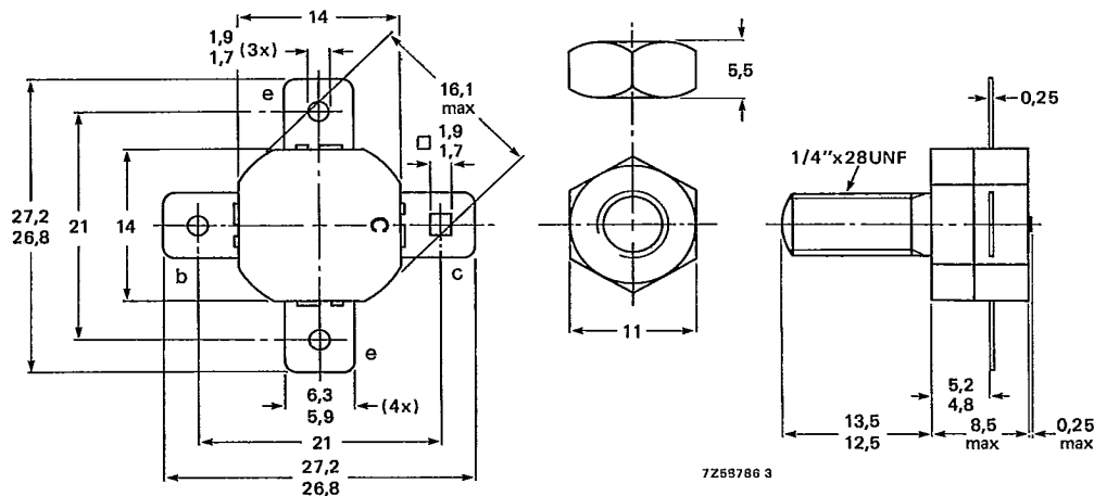
Fig. 1 SOT-55.
